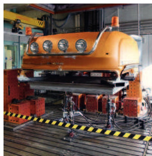
Гидроимпульсный испытательный стенд имитирует выбоины и плохие дорожные условия.
